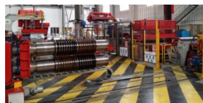
Línea de corte longitudinal con robot de montaje
