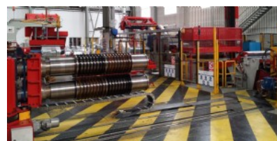
Línea de corte longitudinal con robot de montaje
